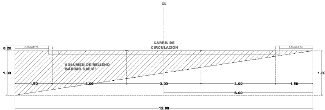
Ilustración 13. Esquema de área de sólo relleno
