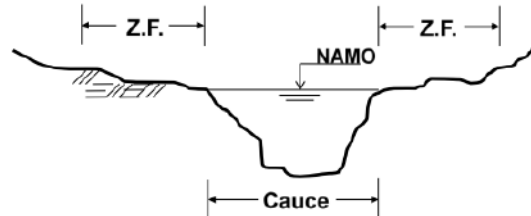
Ilustración 15. Esquema de delimitación de cauce y franjas de zona federal
