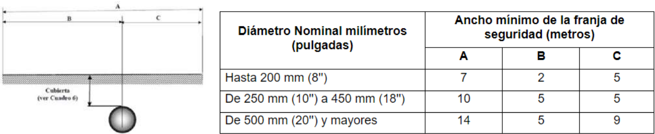
Ilustración 17. Derecho de vía para ductos
