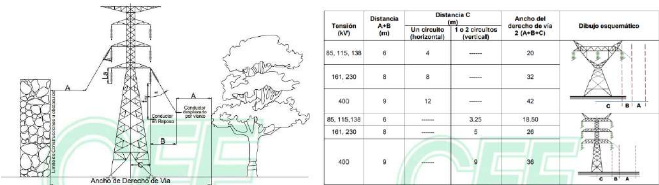
Ilustración 16. Integración de derecho de vía
