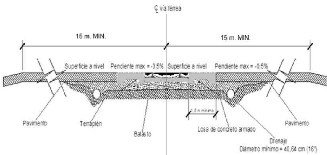
Ilustración 14. Derecho de vía férrea
