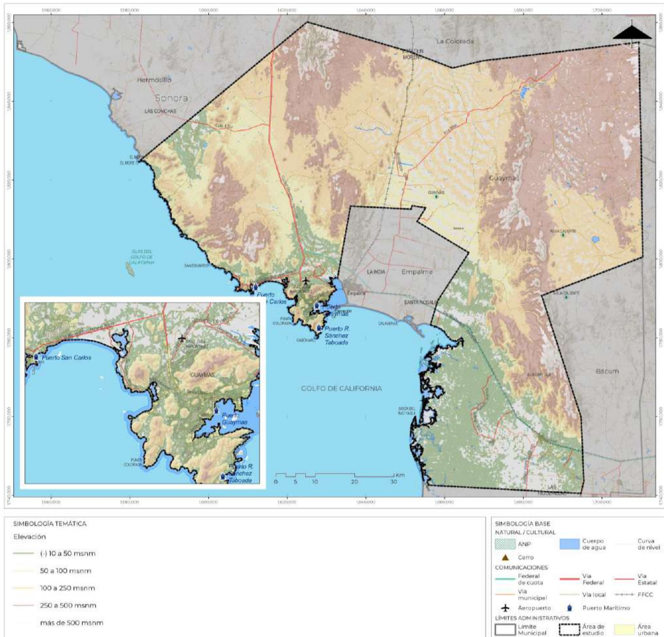
Mapa 2. Hipsométrico Municipio de Guaymas
