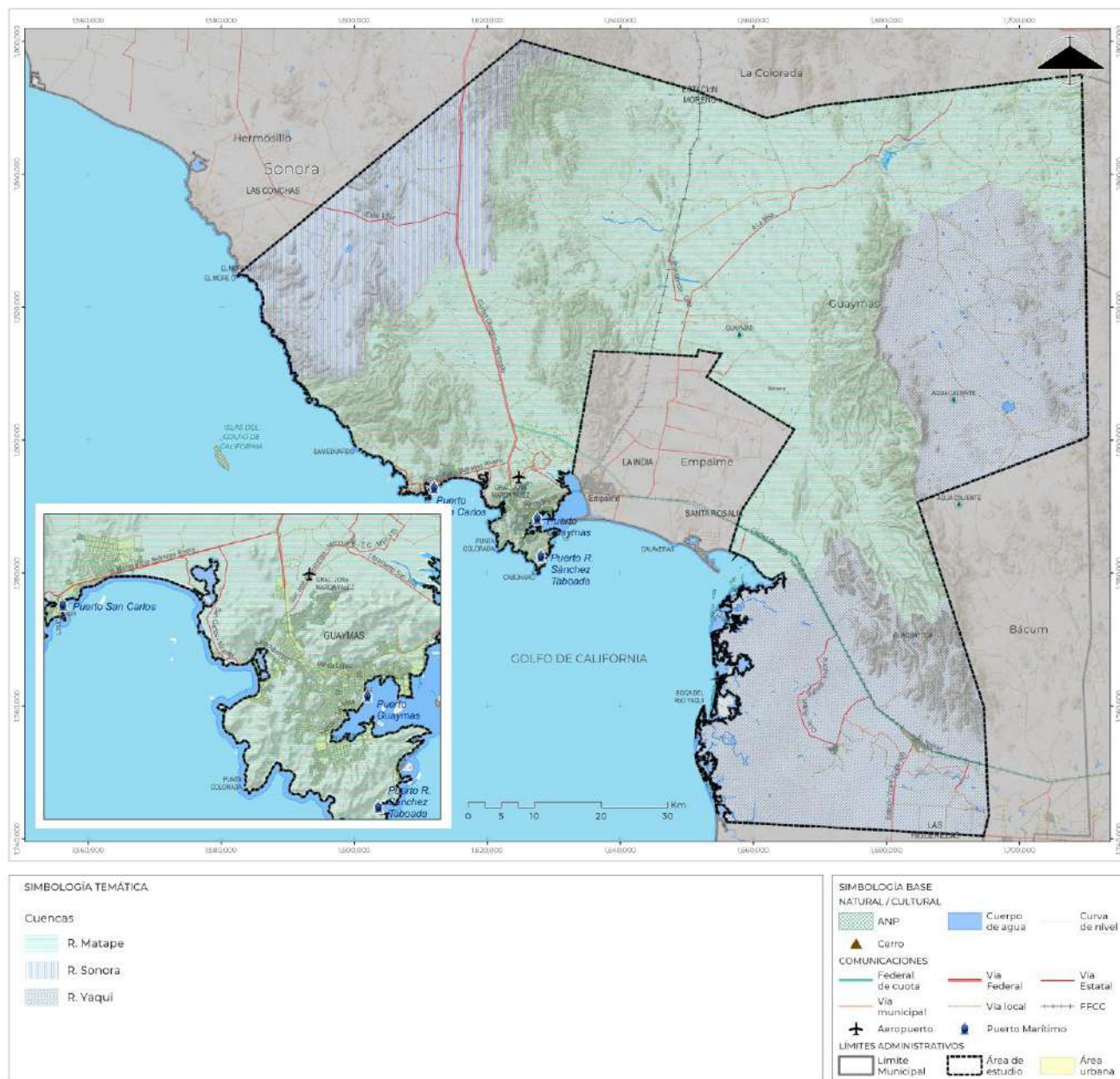
Mapa 3. Cuencas hidrológicas, Municipio de Guaymas
